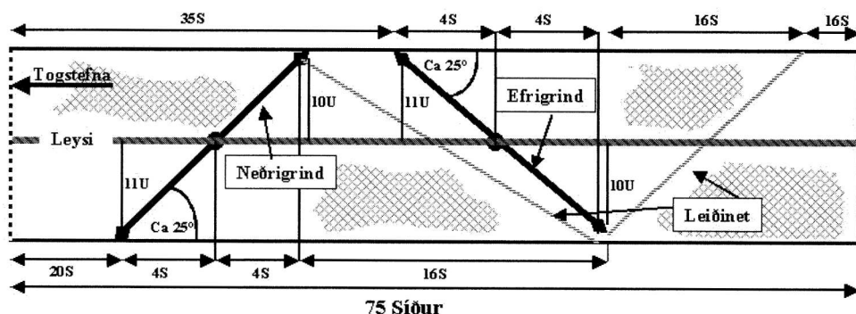
Mynd 3. Staðsetning grinda og leiðineta í skiljunneti.
