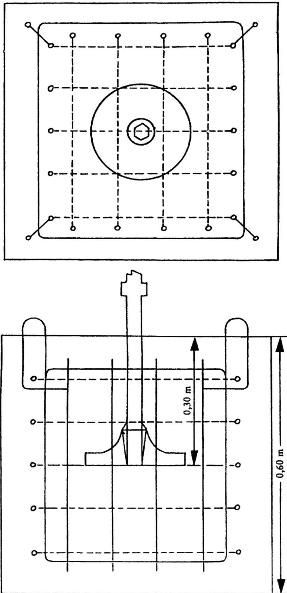
Mynd 10.2 Prófunarklumpur.
