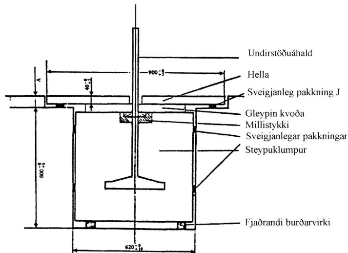
Mynd 10.3 Prófunarbúnaður.
