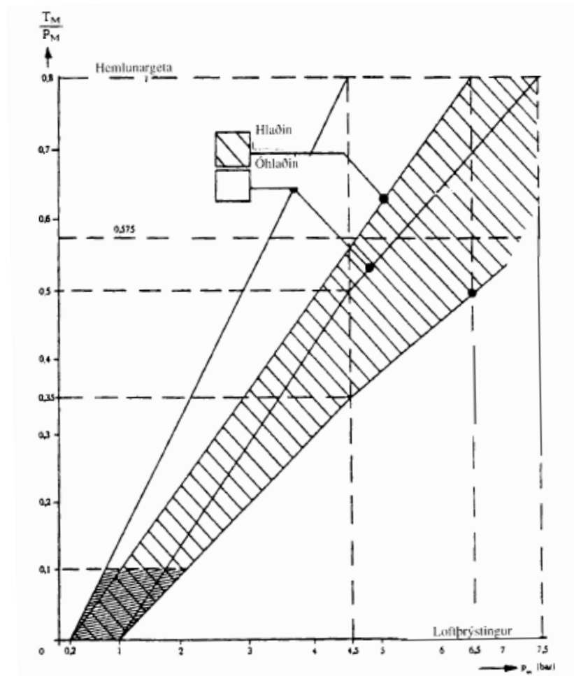
Mynd 6.2: Línurit fyrir dráttarbifreið sem gerð er til að draga festivagn.
