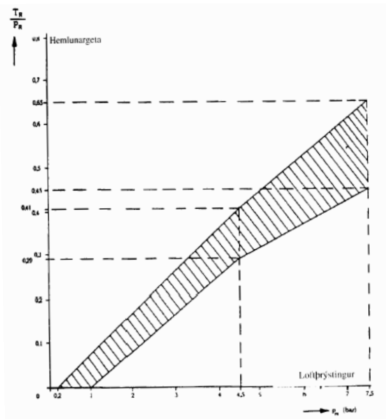
Mynd 6.3: Línurit fyrir festivagn.
